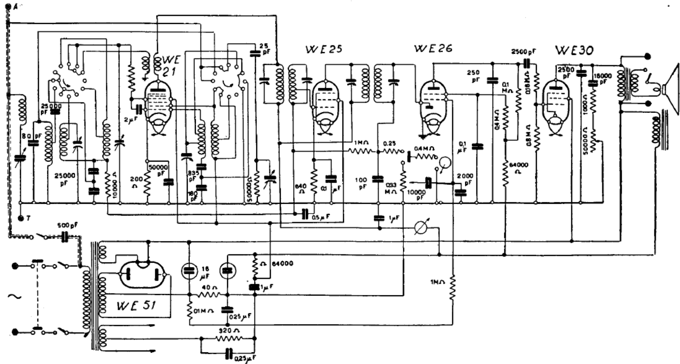
PHILIPS RADIO. — Mod. « 428 » e anche « 651 M, 653 M ». — (SUPER POPE P97A). — Media frequenza: 468 kHz. — Potenza: 3 W. — Produzione: 1935-1936.
